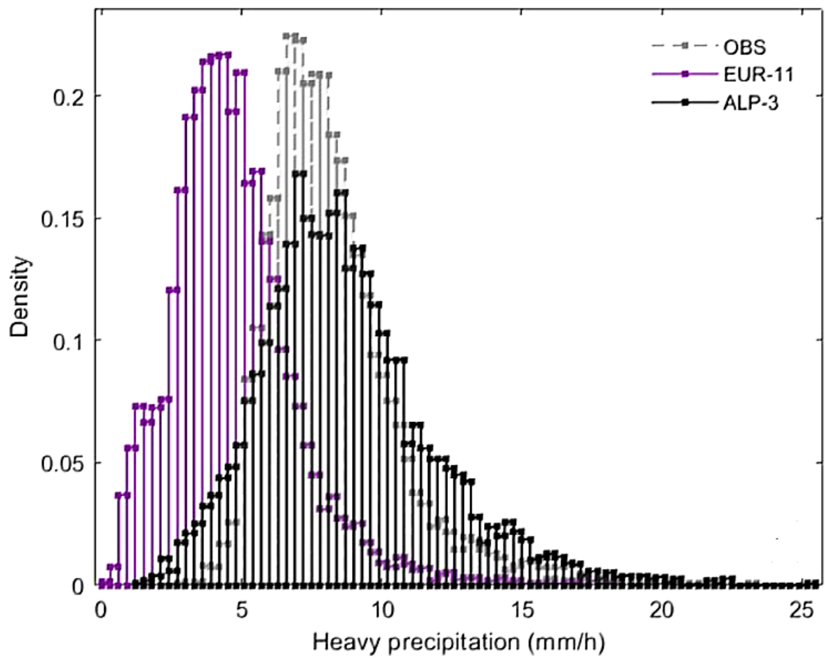
Abbildung 2: Wahrscheinlichkeitsdichte des 99,9 Perzentils des stündlichen Niederschlags im Alpenraum und Süddeutschland für eine konvektionserlaubende Simulation (Schwarz), eine konvektionsparametrisierende Simulation (Lila) und den Beobachtungsdatensatz (Grau) (Adinolfi, Raffa, Reder, & Mercogliano, 2020).
