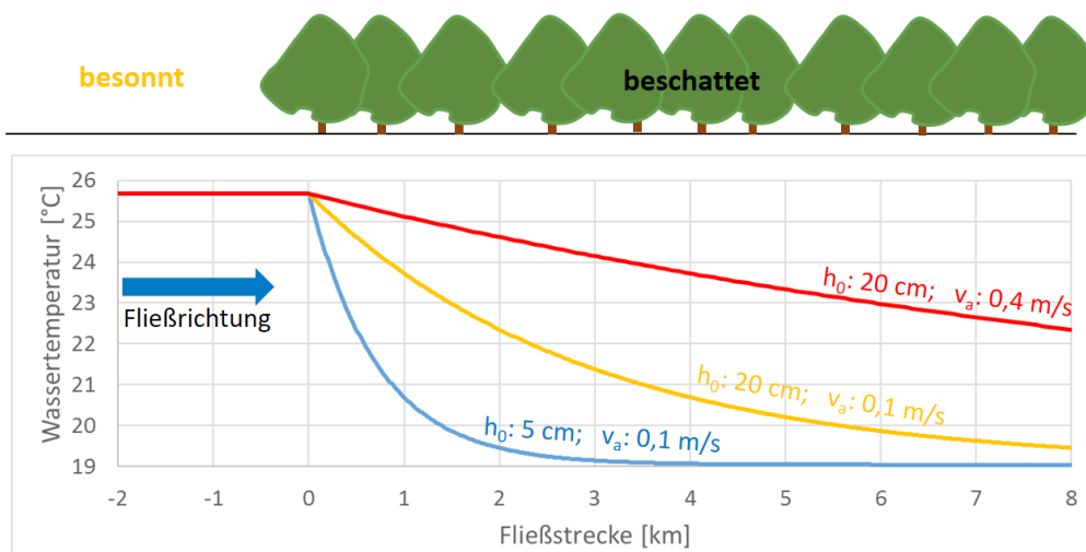
Abbildung 4: Längsverlauf der Wassertemperatur (Tagesmittel) nach dem Übergang von einem besonnten zu einem maximal beschatteten (BI=0,15) Gewässerabschnitt für unterschiedliche Wassertiefen ( h_0 ) und Fließgeschwindigkeiten ( v_a ).
