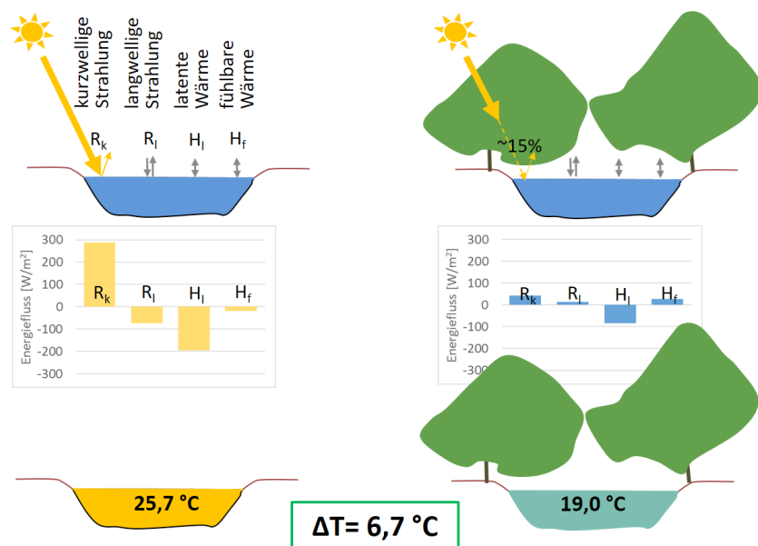
Abbildung 2: Schematische Darstellung der Wirkung dichter Ufervegetation auf die Tagesmittel von Energiebilanz und Wassertemperatur eines schmalen Bachs ( BI=0,15 ) unter charakteristischen meteorologischen Bedingungen eines 1. Augusts (siehe 1. Zeile in Tabelle 1).
