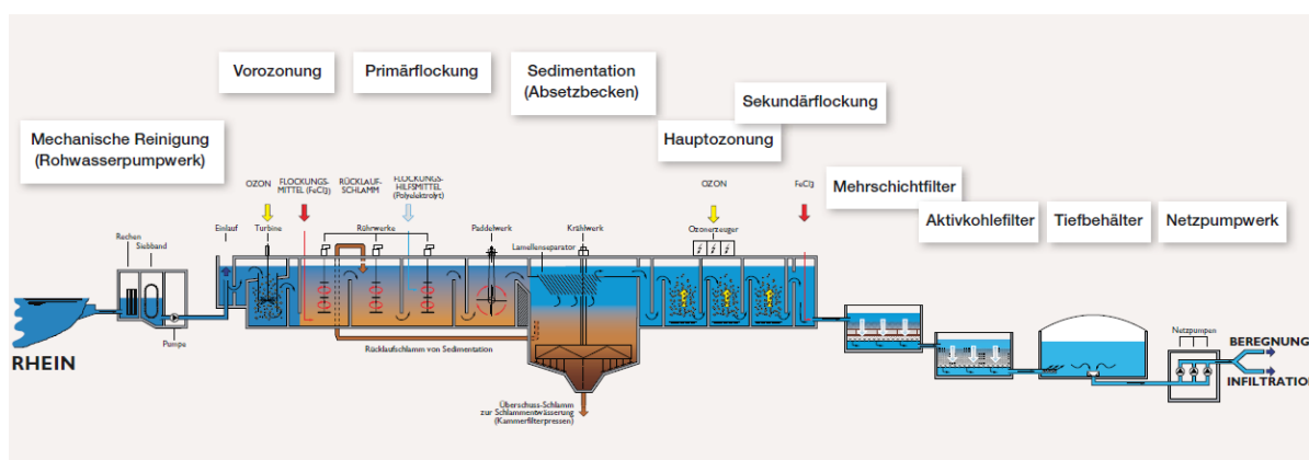
Abbildung 1: Mehrstufiges Aufbereitungsverfahren.
